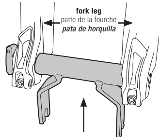
Thru-Axle Adapter adaptateur pour essieu de bord en bord Adaptador para eje pasante
